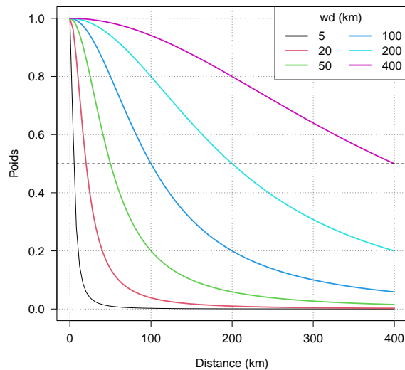
FIGURE 8 – Variation des poids pour différentes valeurs de wd .
