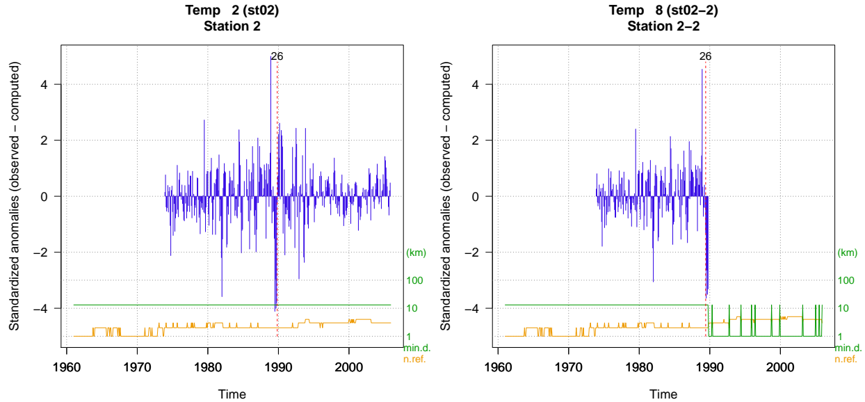
FIGURE 7 – Exemple de détection de sauts dans la moyenne (gauche) et reconstruction des séries à partir de chaque fragment homogène (droite).
